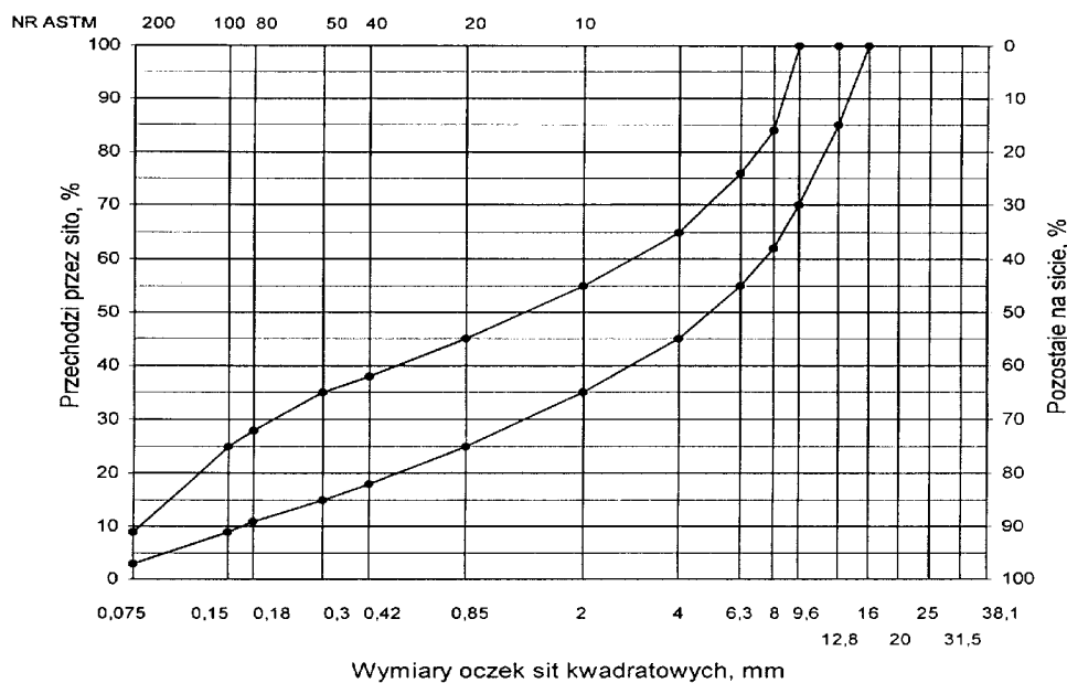
11. Krzywe graniczne uziarnienia mieszanki mineralnej BA od 0 do 25 mm do warstwy wiążącej, wyrównawczej i wzmacniającej nawierzchni drogi o obciążeniu ruchem od KR3 do KR6
