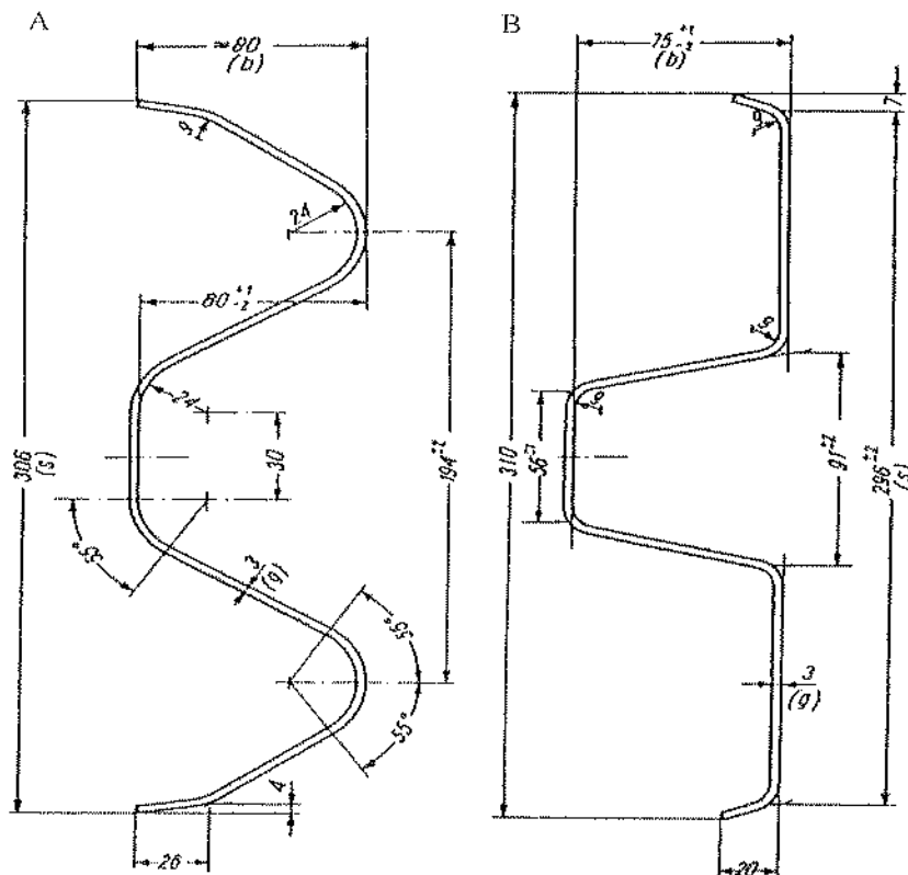
Załącznik 11.4. Profilowana taśma stalowa typu A i B, wg L. Mikołajków: Drogowe bariery ochronne, WKiŁ, 1983
