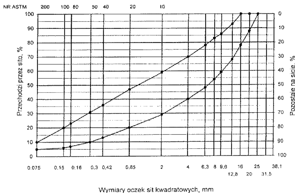
Rys. 1. Krzywe graniczne uziarnienia mieszanki mineralnej BA od 0 do 20 mm do warstwy ścieralnej nawierzchni drogi o obciążeniu ruchem dla KRI lub KR2
